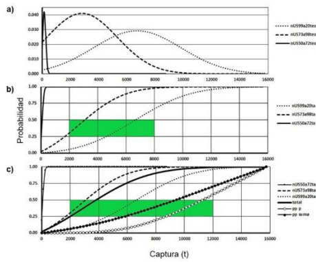
Figura 6. Distribución de los datos de capturas totales normalizadas respecto de sus promedios y desviaciones estándares, panel a) distribuciones en sentido inferencial o de uso común. Panel b) la suma acumulada es 1, en sentido bayesiano. El panel c) lo mismo que en panel b) con los resultados de las probabilidades posteriores obtenidas del producto (pp p) y de la suma (pp suma). Con colores se enfatizan las intersecciones con 0.5 o 50 % de probabilidad o tendencia central.
