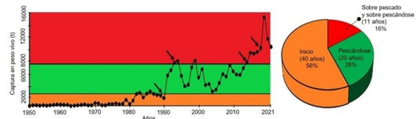
Figura 4. Capturas de pez espada reportados por la FAO (2021), evaluados respecto del percentil de entre el 15 y el 85% de las capturas o del indicador de abundancia. En la gráfica de pastel, se indica el nombre la categoría, el número de años y el porcentaje del total (---- OPO, p 15 continua delgada, p 85 continua gruesa).
