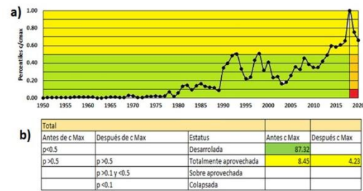
Figura 5. Panel a) datos de las capturas de pez espada en el OPO, reportados por la FAO (2021) evaluados respecto del máximo de las capturas o del indicador de abundancia máximo, organizados en proporciones de c/c_{Max} . Panel b) periodo respecto c/c_{Max} = 1 , el estatus y el porcentaje del total. Se utilizan los términos de aprovechamiento.
