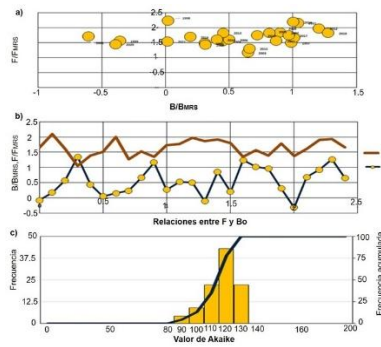
Figura 8. Salidas de los procesos de ajuste para las relaciones de F/F_{MRS} y B/B_{MRS} , en a), se pueden observar valores >0 por año, que pueden ser utilizados o considerados para el análisis. En la parte b), los valores mencionados como series, al igual para considerar aquellos >0 ; en la parte c), los valores de ajuste utilizando el criterio de Akaike. En general cada corrida en este modelo es de al menos 100 veces, n veces, digamos 20 corridas de estas hasta la convergencia de valores de >0 en a).
