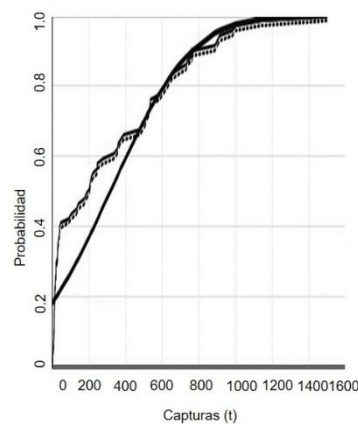
Figura 2. Prueba de normalidad de Kolmogorov-Sminorv, utilizando la diferencia entre probabilidades esperadas y observadas (--- F_0 , --- F_n , - - - F_n - F_0 ).
