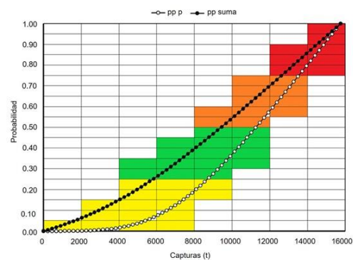
Figura 7. Probabilidades posteriores del producto (pp p) y de la suma (pp suma), obtenida de los datos totales, en tres periodos la serie de tiempo de 1950 a 2020, que fueron de 1950 a 1972, de 1993 a 1998 y de 1999 a 2020 y agrupados. Con colores se enfatizan las intersecciones con 0.5 o 50 % de probabilidad o tendencia central.
