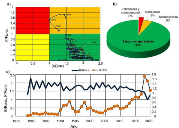
Figura 9. Indicadores de F/F_{MRS} y B/B_{MRS} , después de la n-iteraciones de ajuste, ponderada por años. Panel a) Diagrama de Kobe. Panel b) Porcentaje de participación por fase del diagrama de Kobe. Panel c) Tendencia de F/F_{MRS} y B/B_{MRS} durante la serie de tiempo (1979-2020).
